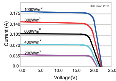
Resultado de la medición de potencia PMP Result of PMP Power Measurement
